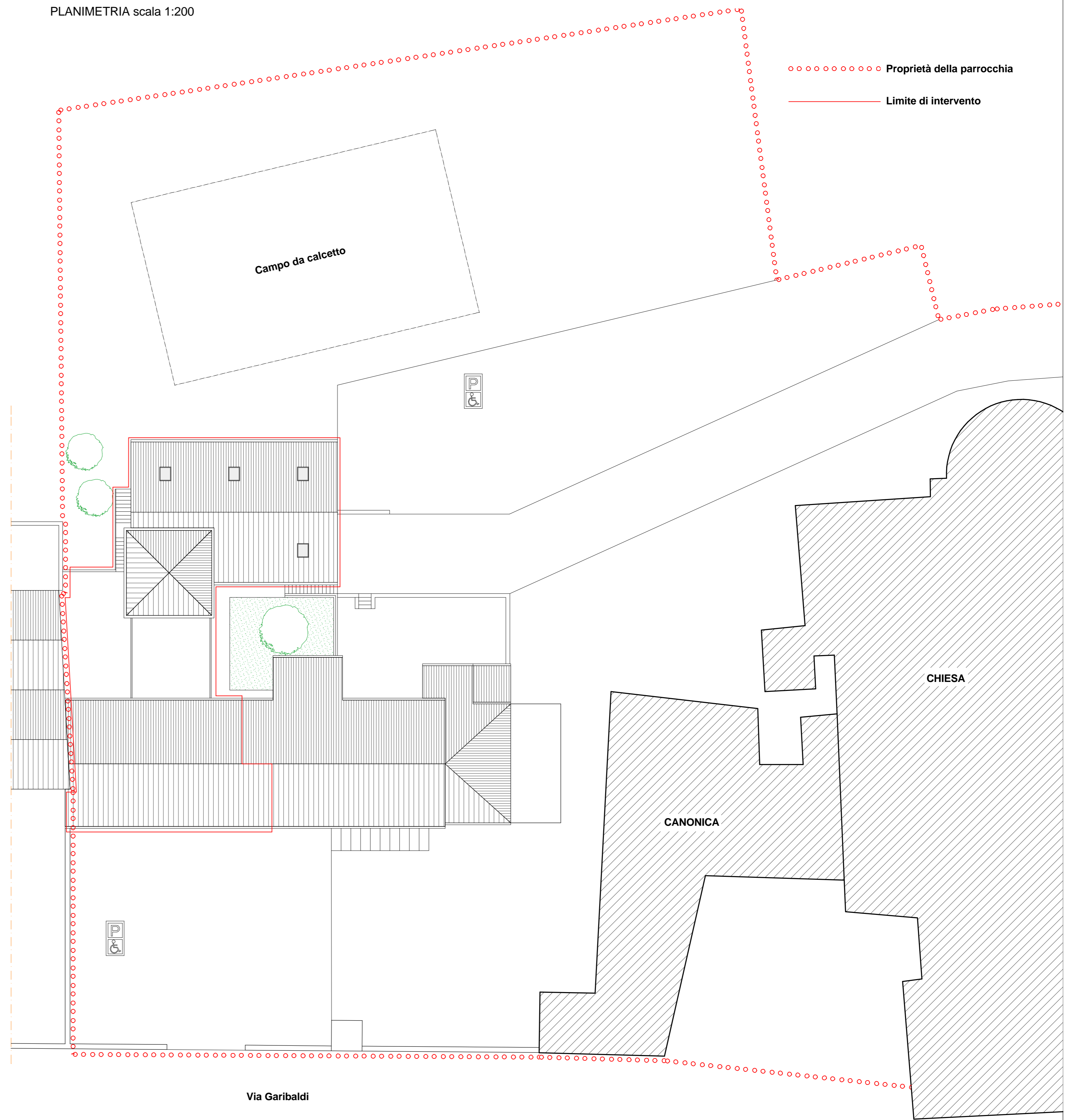
PLANIMETRIA scala 1:200
